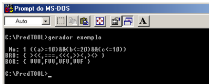
Figura 3.2 – Geração das Restrições Requeridas Pela PredTOOL.
