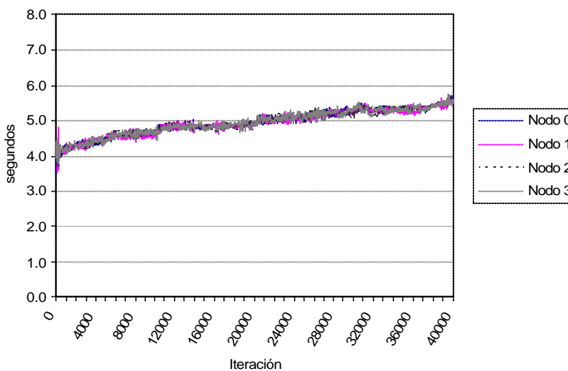
Figura 2. Tiempo de ejecución de cada 20 iteraciones ( T_{actual} ) con Balance de Carga activado con COV=0.02
