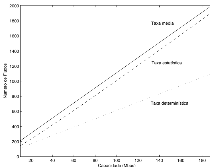
Figure 6: Número de fluxos em função da capacidade do enlace de saída para fluxos do tipo B
