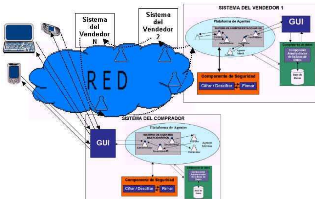
Figura 3. Arquitectura ARAMCEL.
