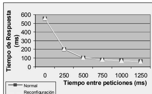
Figura 14. Gráfico de tiempos de lecturas del sistema para el modo normal y en reconfiguración con cargas de científica.
