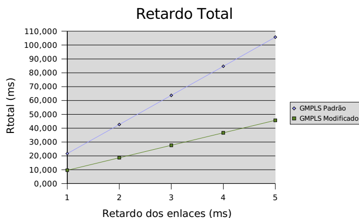
Fig. 4. Retardo Total
