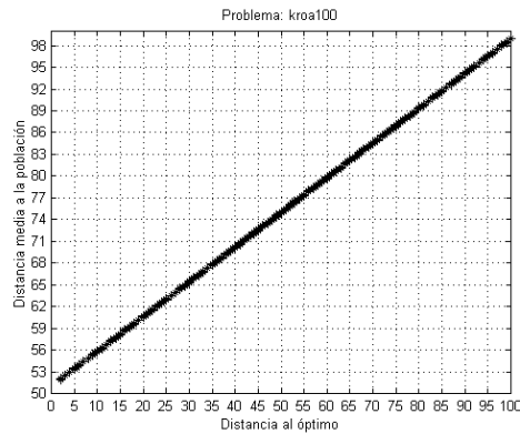
Figura 6.3: \delta(P, r^*) en función de \delta(r, r^*)
