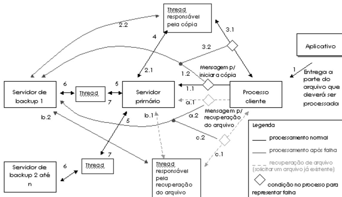
Figura 3.2: Diagrama lógico do sistema de replicação
