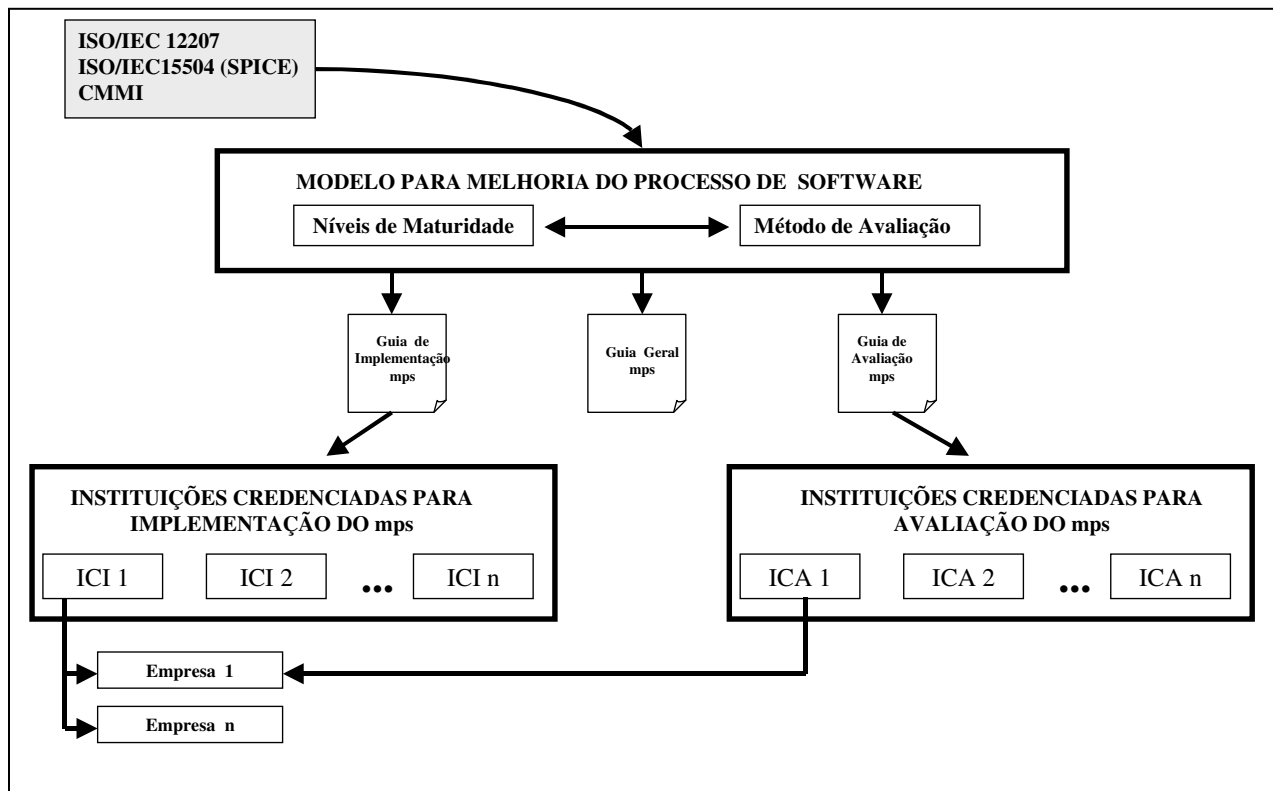
Figura 3 – Modelo de Referência para melhoria do Processo de Software (MR mps)
